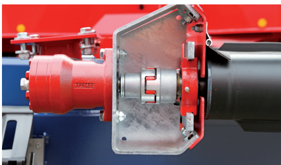
Ajami mootori ja veorulli vahele paigaldatud haakeseadis tagab otseühenduse ja seamete pika tööea.
