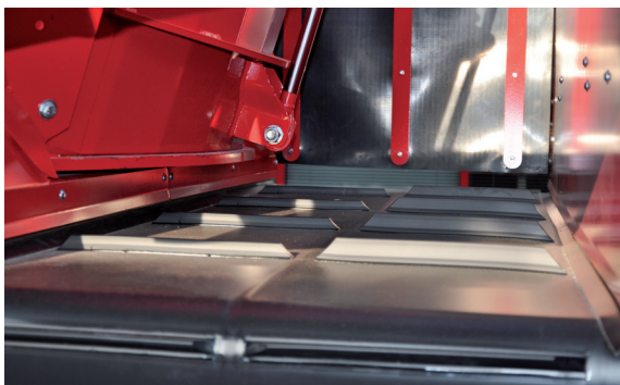
SILOKING ristsuunaline konveierilint ja kokkuvolditav täiendav konveierilint väga kõrgete söödarennide jaoks.
